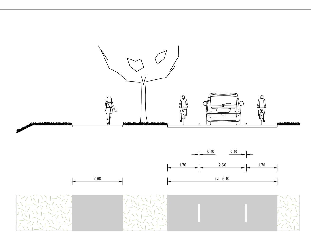
PRINCIEPROFIEL DE ZANDEN SCHAAL 1: 100
